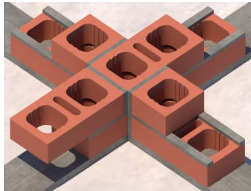
(Encuentro de castillos en "X")
