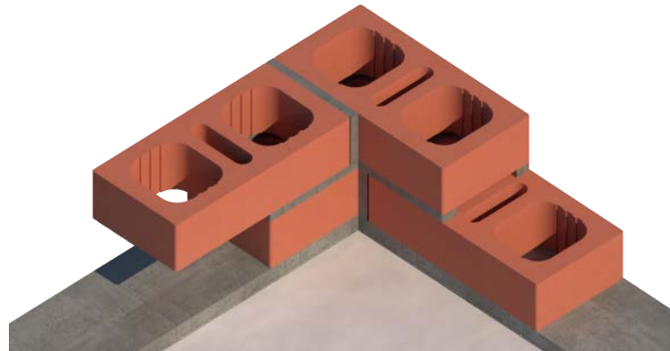
(Encuentro de castillos en "L")
