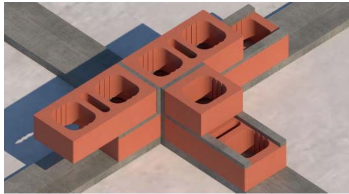
(Encuentro de castillos en "T")
